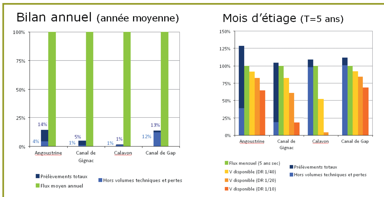
* Bilans besoins/ressource annuels et à l'étiage pour les 4 situations de déséquilibre étudiées.
